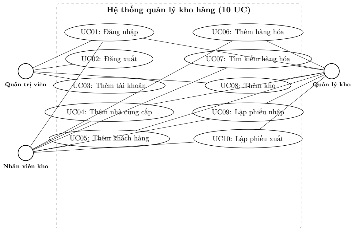
Figure 1: Sơ đồ use case tổng quát (10 use case – mỗi UC một mục tiêu)
